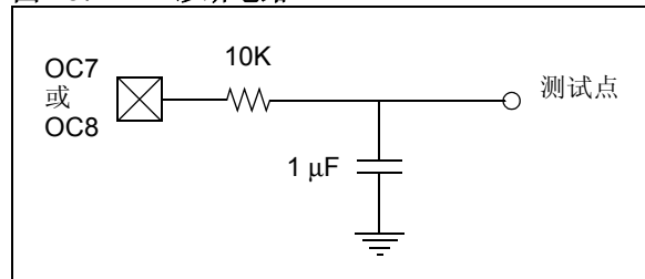
图 13: 诊断电路
