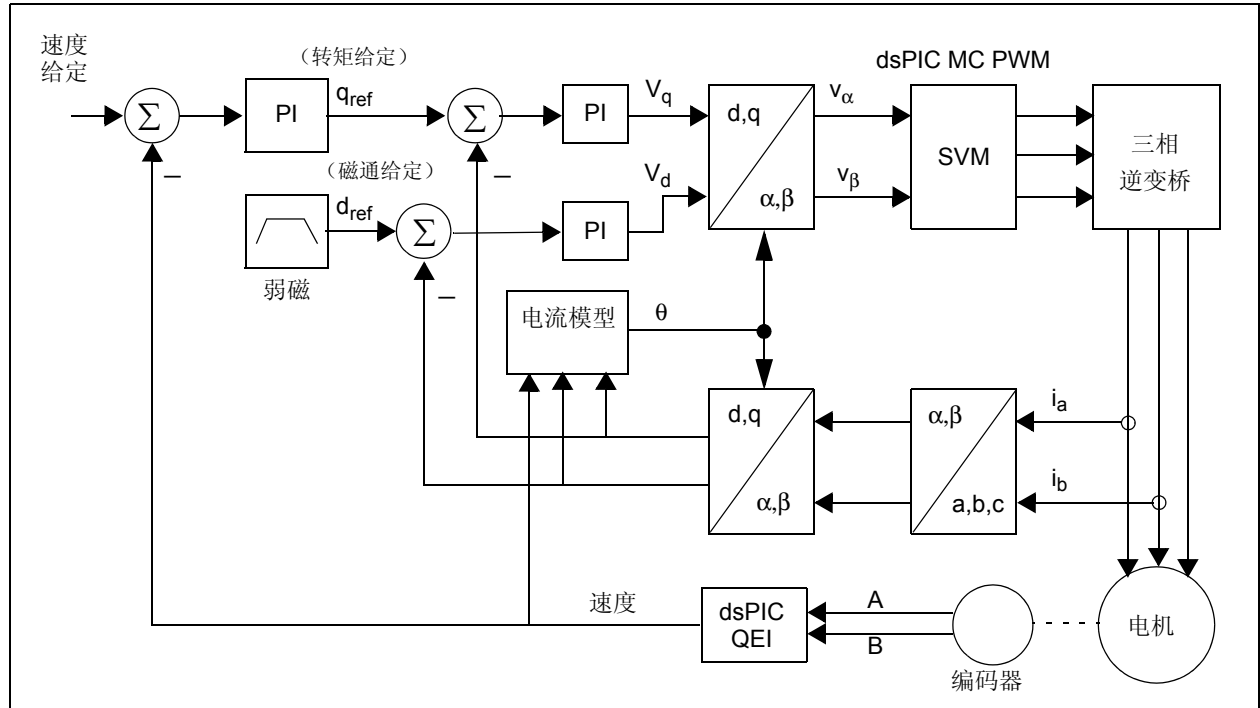
图 1: 矢量控制框图
