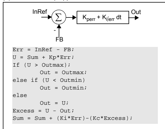
图 6: PI 控制
