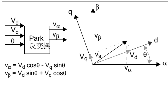
图 4: Park 反变换
