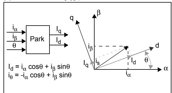
图 3: Park 变换
