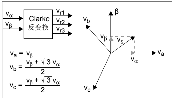
图 5: Clarke 反变换
