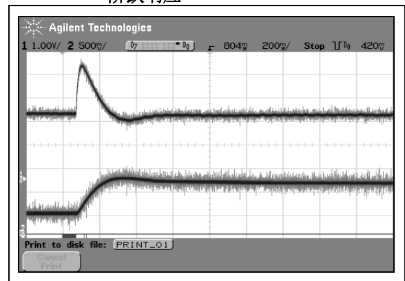
图 14: I_q 与转速，500RPM 至 1000RPM 阶跃响应
