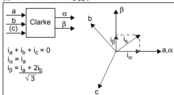
图 2: Clarke 变换
